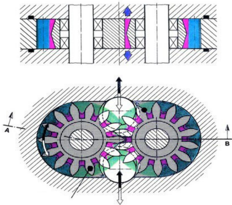
齿轮流量计结构原理图
